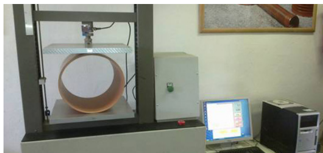
Měření kruhové tuhosti
