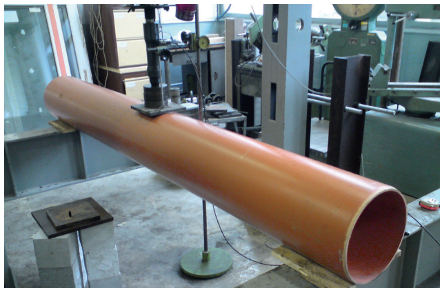
Laboratorní zkouška průhybu
