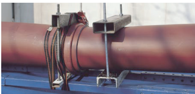
Zkouška těsnosti spoje (PP MASTER)
