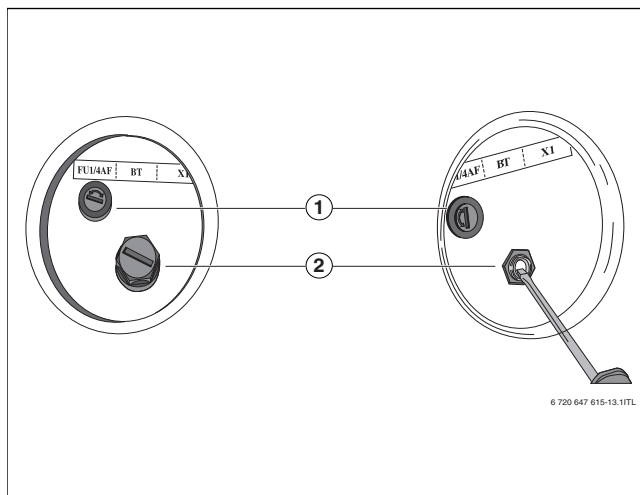
Obr. 3 Odblokování bezpečnostního omezovače teploty (STB)
