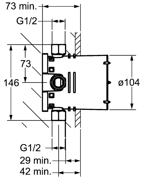
Výkres výrobku
