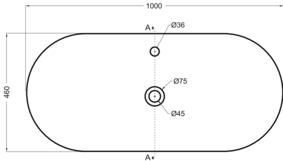
PIANTA PLAN
