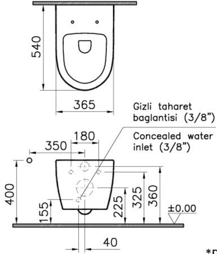
Gizli bağlantı Concealed connection versteckte Verbindung
