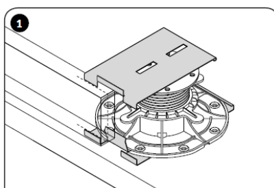
Rozměření na dlažbě
