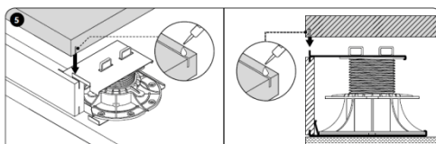
Zámky můžeme prolepit lepidlem
