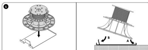
Terč uložíme na spodní profil
