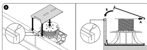
Na hlavu terče uložíme horní profil
