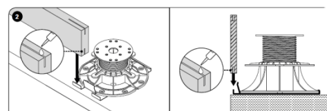
Dle návodu 1 montujeme horizontální profil
