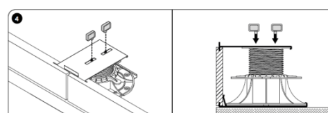
Ve spoji dlažeb montujeme vymezení
