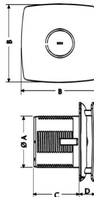
QUICK FIX GRIP (montáž bez vrtání)
