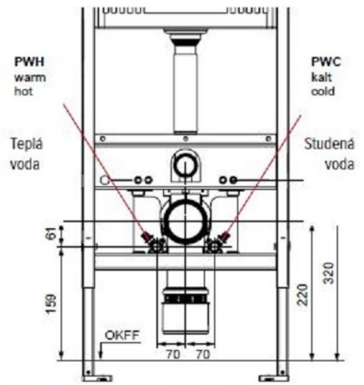
Připojení a rozměry pro sádkartonové příčky
