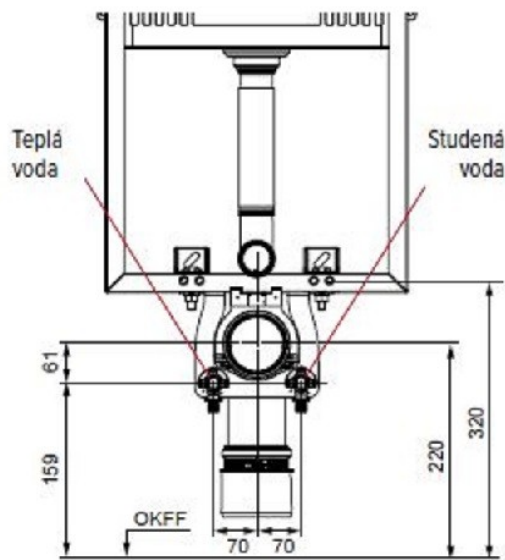
Připojení a rozměry pro zděné příčky
