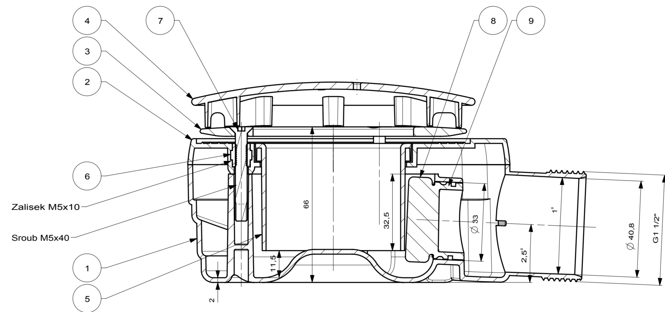
SECTION A-A
