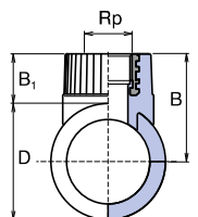
Navarovací sedlo s kovovým závitem vnitřním
