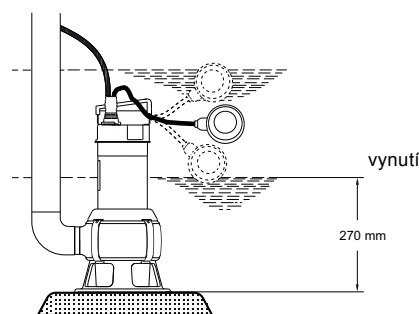
Obr. 5 Nastavení plovákového spínače
