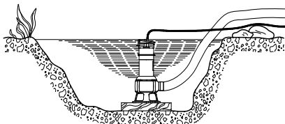
Obr. 4 Umístění čerpadla na pevném základu Čerpadlo nesmí být zavěšeno na výtlačném potrubí.
