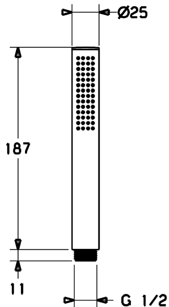
Výkres výrobku
