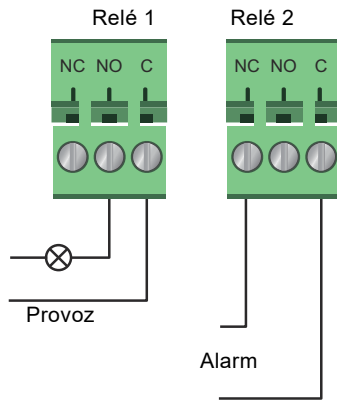
Obr. 46 Releový výstup
