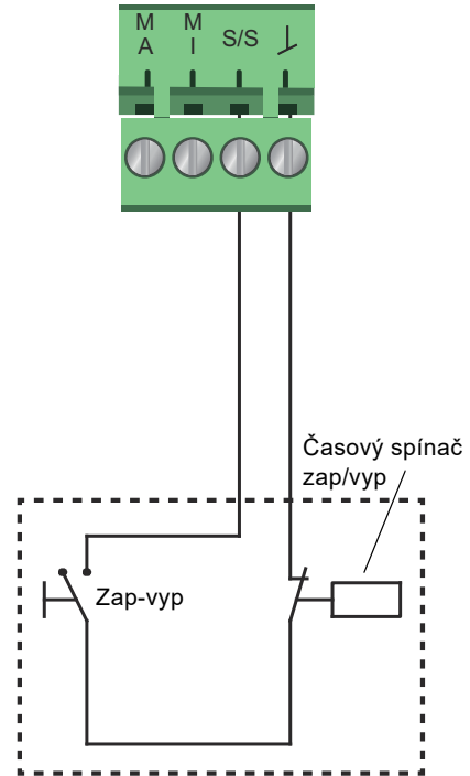
Obr. 47 Digitální vstup
