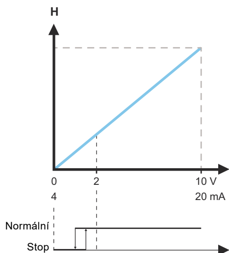
Obr. 56 "Lineární se stop", 0-10 V
