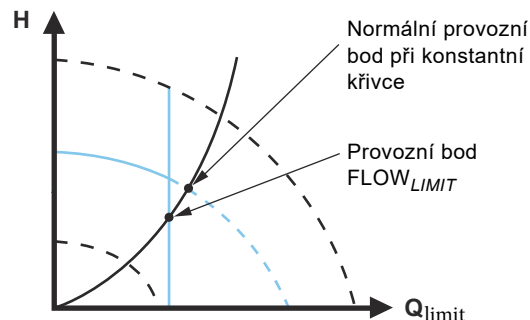
Obr. 41 Konstantní křivka pomocí funkce FLOW LIMIT
