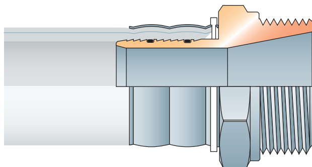
Průřez zalisovanou kovovou tvarovkou 40 - 50 mm se zalisovanou objímkou z nerezové oceli
