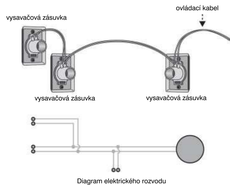
Zapojení zásuvek v sérii
