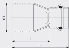
Prestabo-redukce - nelegovaná ocel, pozinkováno model 1115.1
