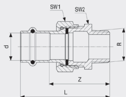
Prestabo-přechodové šroubení - nelegovaná ocel, pozinkováno model 1165
