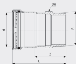
Prestabo-přechodový kus - nelegovaná ocel, pozinkováno model 1111
