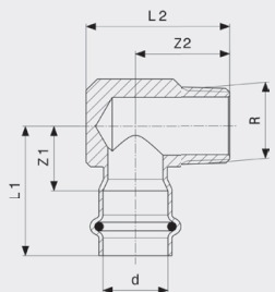
Prestabo-přechodové koleno 90° - nelegovaná ocel, pozinkováno model 1114.1
