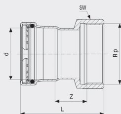
Prestabo XL-přechodový kus - nelegovaná ocel, pozinkováno model 1112XL
