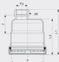
Prestabo XL-víčko - nelegovaná ocel, pozinkováno model 1156XL
