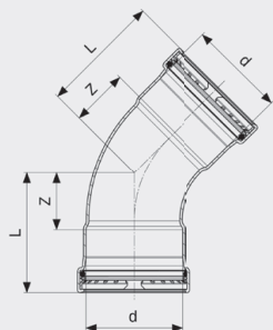
Prestabo XL-oblouk 45° - nelegovaná ocel, pozinkováno model 1126XL
