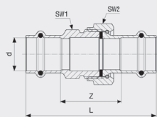
Prestabo-šroubení - nelegovaná ocel, pozinkováno model 1160
