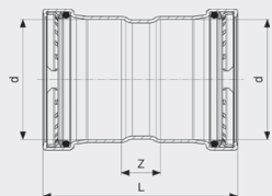
Prestabo XL-objímka - nelegovaná ocel, pozinkováno model 1115XL
