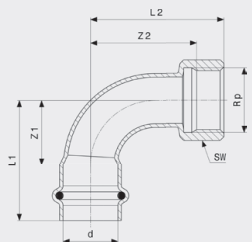
Prestabo-přechodový oblouk 90° - nelegovaná ocel, pozinkováno model 1114.5
