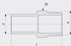
Prestabo-zásuvný kus - nelegovaná ocel, pozinkováno model 1111.1
