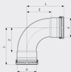
Prestabo XL-oblouk 90° - nelegovaná ocel, pozinkováno model 1116XL
