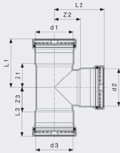
Prestabo XL-T-kus - nelegovaná ocel, pozinkováno model 1118XL
