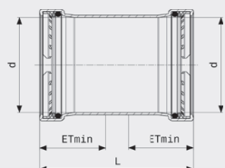
Prestabo XL-posuvná objímka - nelegovaná ocel, pozinkováno model 1115.5XL
