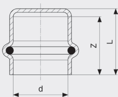
Prestabo-víčko - nelegovaná ocel, pozinkováno model 1156
