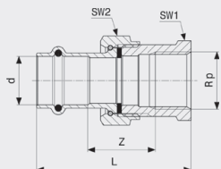
Prestabo-přechodové šroubení - nelegovaná ocel, pozinkováno model 1162
