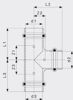
Prestabo-T-kus - nelegovaná ocel, pozinkováno model 1118
