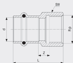
Prestabo-přechodový kus - nelegovaná ocel, pozinkováno model 1112
