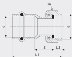
Prestabo-připojovací šroubení - nelegovaná ocel, pozinkováno model 1163
