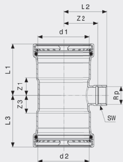
Prestabo XL-T-kus - nelegovaná ocel, pozinkováno model 1117.2XL
