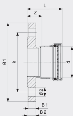
Prestabo XL-přírubový přechod - nelegovaná ocel, pozinkováno model 1159XL
