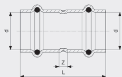
Prestabo-objímka - nelegovaná ocel, pozinkováno model 1115
