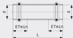
Prestabo-posuvná objímka - nelegovaná ocel, pozinkováno model 1115.5
