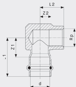
Prestabo-přechodové koleno 90° - nelegovaná ocel, pozinkováno model 1114.2
