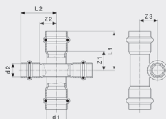
Prestabo-křížová tvarovka - nelegovaná ocel, pozinkováno model 1148
