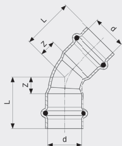
Prestabo-oblouk 45° - nelegovaná ocel, pozinkováno model 1126
