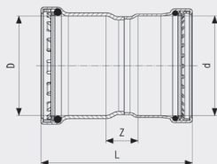
Megapress S XL-přechodový kus - nelegovaná ocel, povrchová úprava zinkem a niklem model 4213XL
