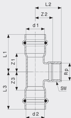
Prestabo-T-kus - nelegovaná ocel, pozinkováno model 1117.2
