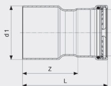
Prestabo XL-redukce - nelegovaná ocel, pozinkováno model 1115.1XL
