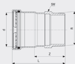
Prestabo XL-přechodový kus - nelegovaná ocel, pozinkováno model 1111XL
