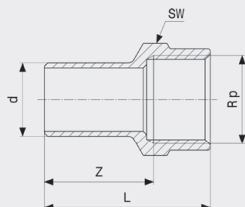
Prestabo-zásuvný kus - nelegovaná ocel, pozinkováno model 1112.1
