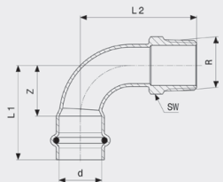
Prestabo-přechodový oblouk 90° - nelegovaná ocel, pozinkováno model 1114
