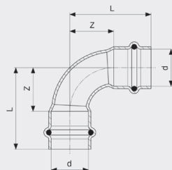
Prestabo-oblouk 90° - nelegovaná ocel, pozinkováno model 1116
