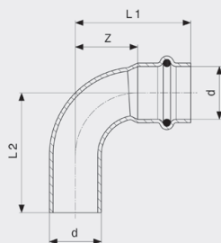
Prestabo-oblouk 90° - nelegovaná ocel, pozinkováno model 1116.1
