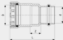
Megapress-přechodový kus - nelegovaná ocel, povrchová úprava zinkem a niklem model 4213
