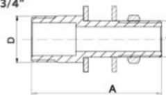
FT214 Prodloužení do bytového jádra 1/2" x 3/4"
