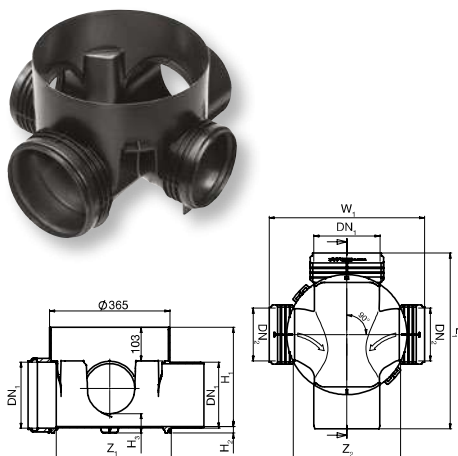
Šachtové dno z PP včetně těsnění – typ III (sběrné 90°)
