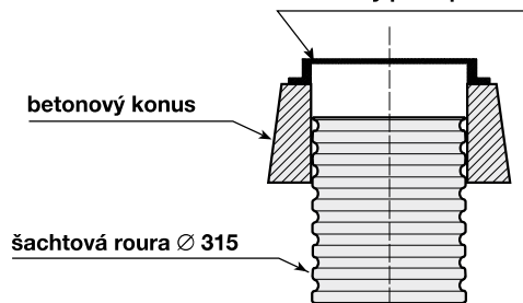
4. Litinový poklop B125
