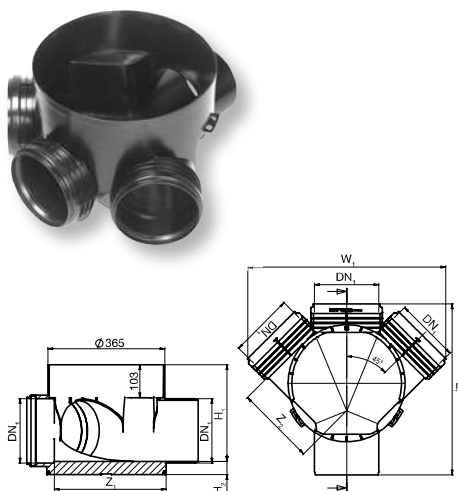
Šachtové dno z PP včetně těsnění – typ II (sběrné 45°)
