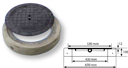
Litinový poklop B125 Ø 400 mm – s betonovým rámem / do šachtové roury
