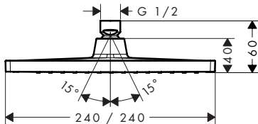
Crometta E 240 1jet 26726XX0 / 26726005 Crometta E 240 1jet Eco 26727XXX
