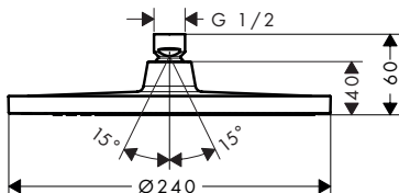
Crometta S 240 1jet 26723XXX Crometta S 240 1jet Eco 26724XXX
