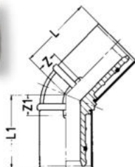
M-press – Koleny 45°
