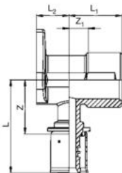
M-press – Nástěnné koleno 90° – vnitřní závit
