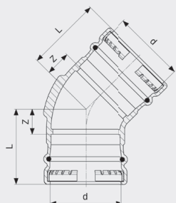
Sanpress XL-oblouk 45° - červený bronz model 2226XL
