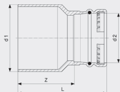
Sanpress XL-redukční kus - červený bronz model 2215.1XL
