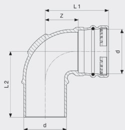
Sanpress-oblouk 90° - červený nebo křemíkový bronz model 2216.1
