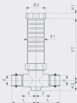
Easytop-podomítkový přímý ventil model 2278.5
