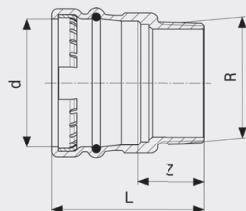
Sanpress XL-přechodový kus - červený bronz model 2211XL
