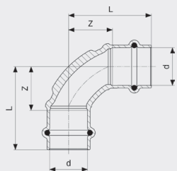
Sanpress-oblouk 90° - červený nebo křemíkový bronz model 2216
