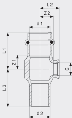
Sanpress-T-kus, G¼, se zásuvným koncem - červený nebo křemíkový bronz model 2217.4
