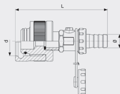
Odtlačovací zátká - mosaz model 2269
