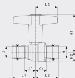
Easytop-kulový kohout model 2275
