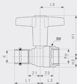
Easytop-kulový kohout model 2275.4
