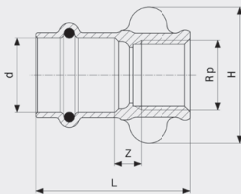
Sanpress-přechodový kus - červený nebo křemikový bronz model 2212.3
