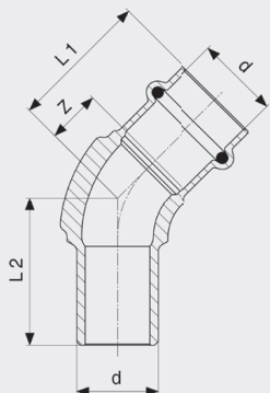
Sanpress-oblouk 45° - červený nebo křemíkový bronz model 2226.1
