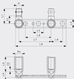
Sanpress-montážní jednotka model 2221.1
