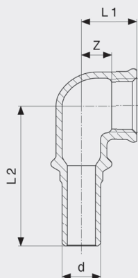
Sanpress-zásuvné koleno 90° - červený nebo křemíkový bronz model 2214.3
