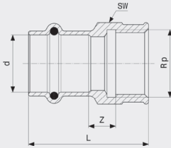
Sanpress-přechodový kus - červený nebo křemikový bronz model 2212
