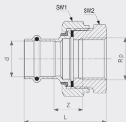
Sanpress-izolační šroubení - červený nebo křemikový bronz model 2267
