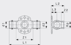
Sanpress-nástěnný T-kus - červený nebo křemíkový bronz model 2217.3
