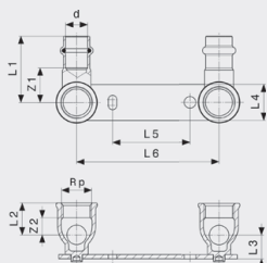
Sanpress-montážní jednotka model 2222.2
