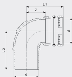
Sanpress XL-oblouk 90° - červený bronz model 2216.1XL
