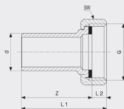
Sanpress-připojovací šroubení - červený nebo křemikový bronz model 2264
