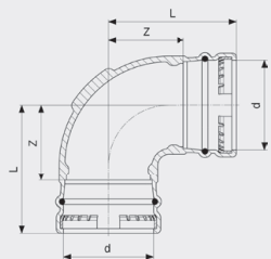
Sanpress XL-oblouk 90° - červený bronz model 2216XL
