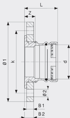
Sanpress XL-přírubový přechod - červený bronz model 2259.3XL
