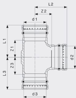
Sanpress XL-T-kus - červený bronz model 2218XL
