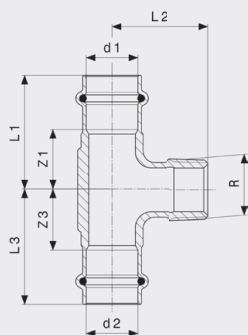
Sanpress-T-kus - červený nebo křemikový bronz model 2217.1
