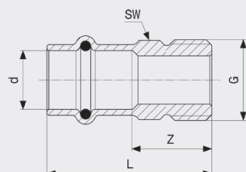
Sanpress-přechodový kus - červený nebo křemíkový bronz model 2211.4
