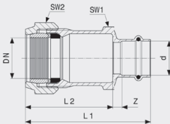
Sanpress-přechodové šroubení - červený nebo křemikový bronz model 2215.6
