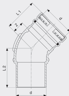
Sanpress XL-oblouk 45° - červený bronz model 2226.1XL
