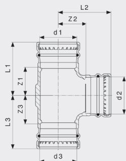
Sanpress-T-kus - červený nebo křemíkový bronz model 2218
