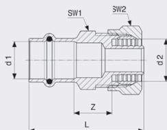
Sanpress-přechodové šroubení - červený bronz model 2213
