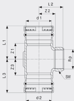
Sanpress XL-T-kus - červený bronz model 2217.2XL
