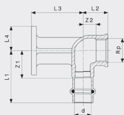
Sanpress-nástěnka - červený nebo křemíkový bronz model 2225.6
