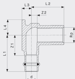
Sanpress-nástěnka - červený nebo křemíkový bronz model 2225
