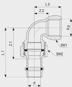
Sanpress-přechodové šroubení 90° - červený nebo křemíkový bronz model 2255
