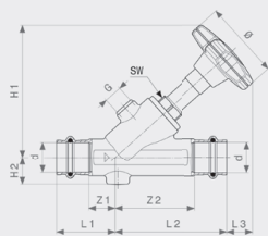
Easytop-ventil se šikmým sedlem model 2237.5
