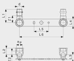
Sanpress-montážní jednotka model 2222.05
