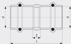
Sanpress-objímka - červený nebo křemíkový bronz model 2215
