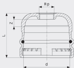
Sanpress XL-vívko - červený bronz model 2256XL
