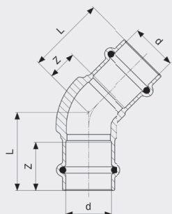
Sanpress-oblouk 45° - červený nebo křemíkový bronz model 2226
