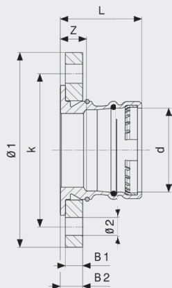
Sanpress XL-přírubový přechod - červený bronz model 2259.5XL
