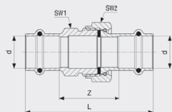
Sanpress-šroubení - červený nebo křemíkový bronz model 2260
