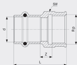
Profipress G-přechodový kus - červený bronz model 2612
