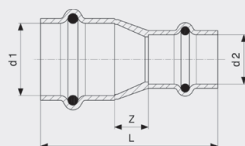
Profipress G-redukovaná objímka - měď model 2615.2
