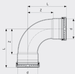
Profipress G XL-oblouk 90° - měď model 2616XL
