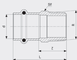
Profipress G-přechodový kus - červený bronz model 2611
