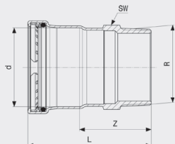
Profipress G XL-přechodový kus - měď model 2611XL
