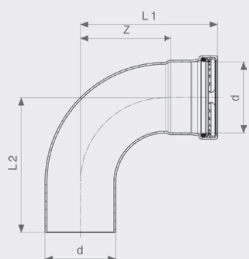
Profipress G XL-oblouk 90° - měď model 2616.1XL
