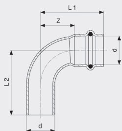
Profipress G-oblouk 90° - měď model 2616.1
