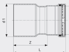
Profipress G XL-redukční kus - měď model 2615.1XL
