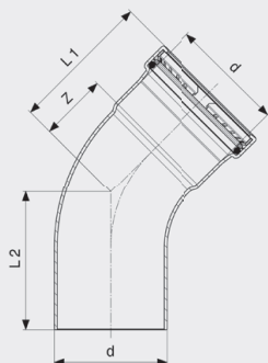
Profipress G XL-oblouk 45° - měď model 2626.1XL
