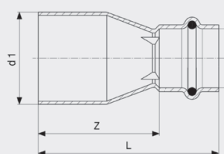
Profipress G-redukční kus - měď model 2615.1
