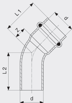
Profipress G-oblouk 45° - měď model 2626.1
