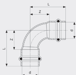
Profipress G-oblouk 90° - měď model 2616
