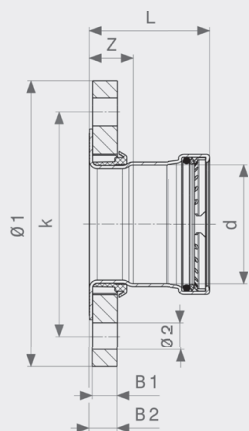
Profipress G XL-přirubový přechod - měď model 2659.5XL
