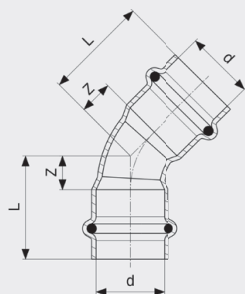
Profipress G-oblouk 45° - měď model 2626
