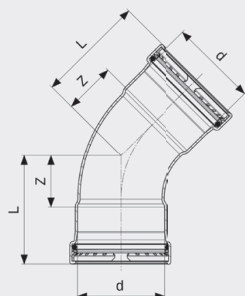
Profipress G XL-oblouk 45° - měď model 2626XL
