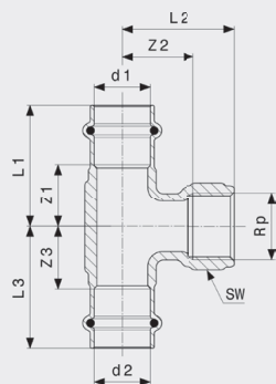
Profifress G-T-kus - červený bronz model 2617.2
