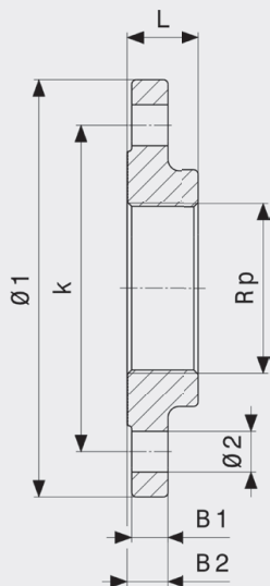
Sanpress XL-příruba, PN 16 - červený bronz model 2259.2XL
