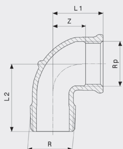
Oblouk 90° - červený bronz model 3092
