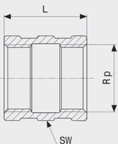
Objímka - červený bronz model 3270
