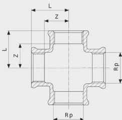
Křížová tvarovka - červený bronz model 3180
