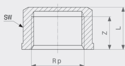
Víčko - červený bronz model 3301
