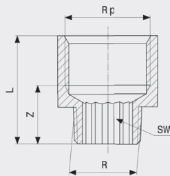
Redukce - červený bronz model 3242
