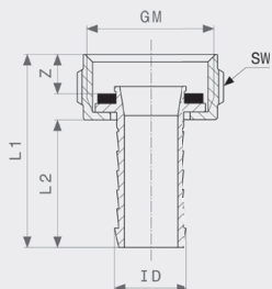
Hadicové šroubení - mosaz model 1811
