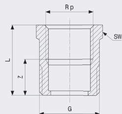
Přechodová vsuvka - červený bronz model 3244
