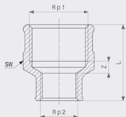
Redukční objímka - červený bronz model 3240
