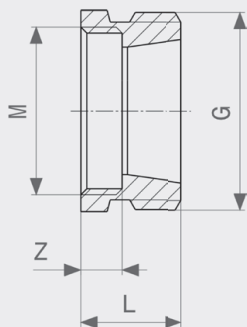
Přechodová vsuvka - červený bronz model 3251
