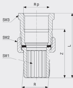
Šroubení - červený bronz model 3331
