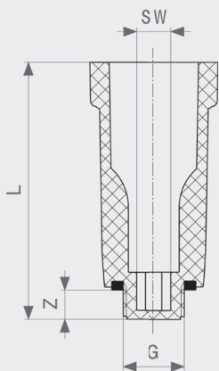
Odtlačovací zátka - plast model 1516
