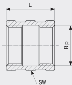
Objímka - červený bronz model 3270
