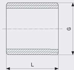
Vsuvka - červený bronz model 3531
