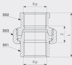
Šroubení - červený bronz model 3340
