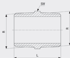
Dvojitá vsuvka - červený bronz model 3280
