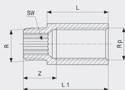
Prodloužení - červený bronz model 3525
