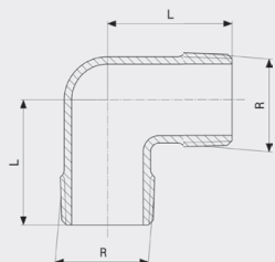
Koleno 90° - červený bronz model 3091
