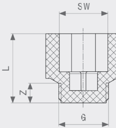
Odtlačovací zátka - plast model 1516.512
