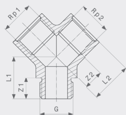
Dvojité připojovací kus - mosaz model 1641
