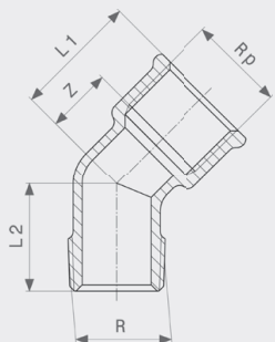
Oblouk 45° - mosaz model 1615
