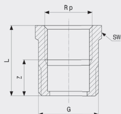
Přechodová vsuvka - červený bronz model 3244
