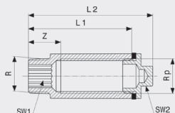
Prodloužení kohoutu - červený bronz model 3527
