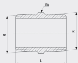
Dvojitá vsuvka - červený bronz model 3280
