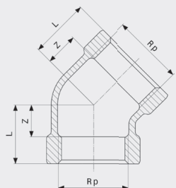
Oblouk 45° - červený bronz model 3120
