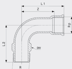
Oblouk 90° - červený bronz model 3001
