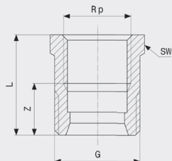
Přechodová vsuvka - červený bronz model 3243
