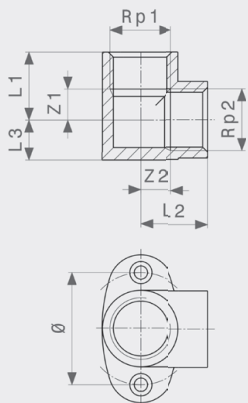
Nástěnka - mosaz model 1421
