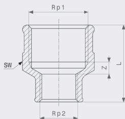
Redukční objímka - červený bronz model 3240
