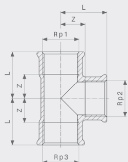
T-kus - mosaz model 1622
