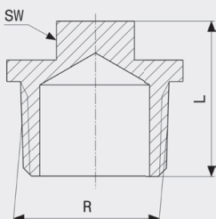
Zátka - červený bronz model 3290
