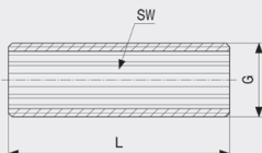
Dlouhá vsuvka - červený bronz model 3535
