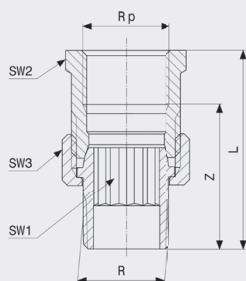
Šroubení - červený bronz model 3341
