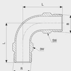
Oblouk 90° - červený bronz model 3003
