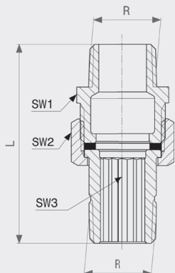
Šroubení - červený bronz model 3334
