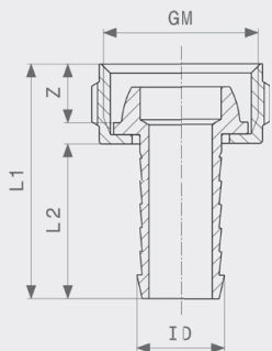
Hadicové šroubení - mosaz model 1812
