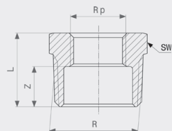
Redukce - červený bronz model 3241
