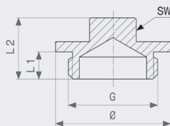
Zátka - mosaz model 1751
