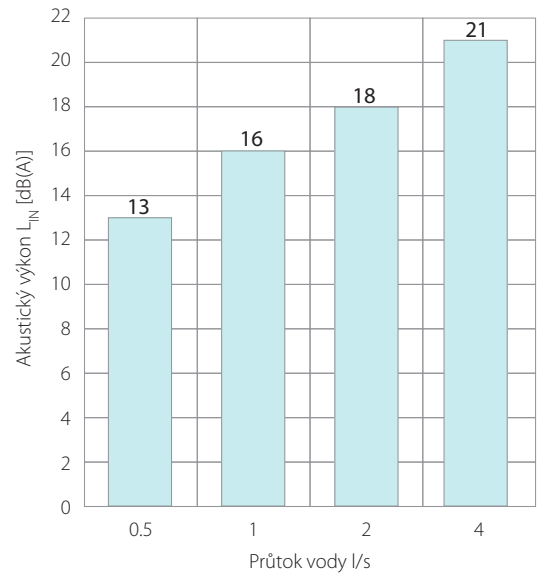
Ultra Silent™ Tlumení hluku L_{IN} DIN 4109
