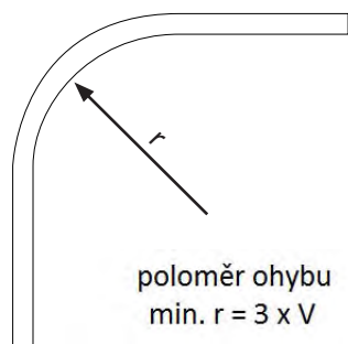
Maximální ohyb vertikální
