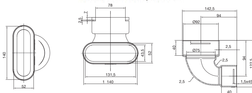
Přechod 90 na Flat 51, Koleno 90°
