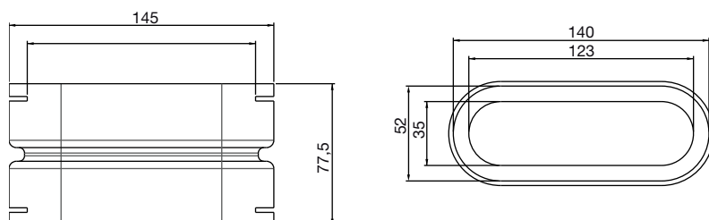
Spojka flat 51
