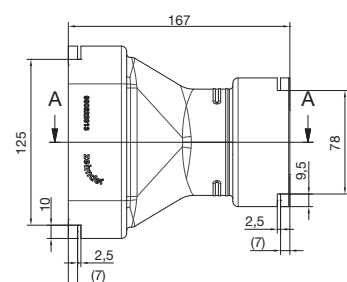
Přechod 90/75 na Flat 51
