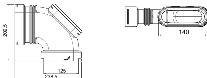
Koleno flat 51 V
