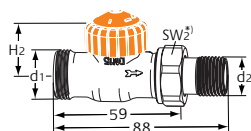
Přímé s vnějším závitem G3/4
