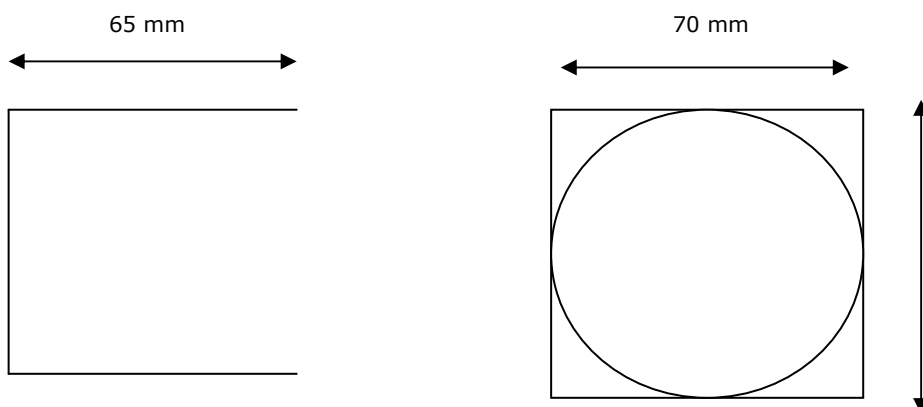
Obr. 5 Otvor ve stěně pro namontování instalační krabice pro regulátor
